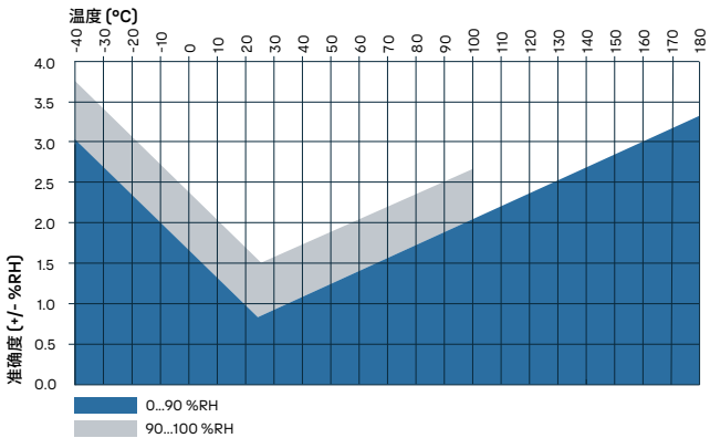
湿度测量精度与温度呈函数关系
