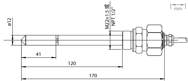
HMP374 尺寸
