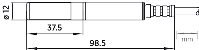
HMP373 尺寸
