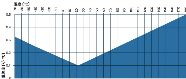
全量程温度测量精度
