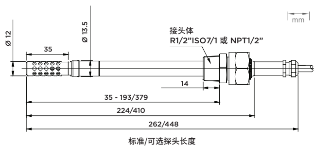
HMP378 尺寸
