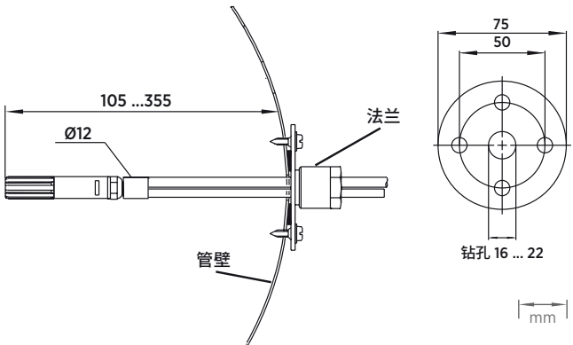
左侧：管道安装套件尺寸。右侧：安装法兰尺寸。铝或不锈钢材质。
