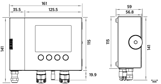
HMT370EX 变送器尺寸
