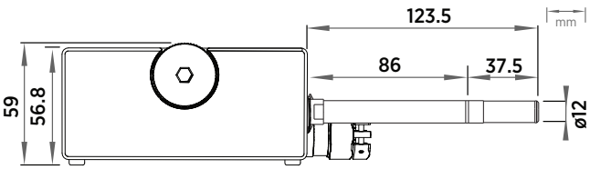
HMP371 尺寸
