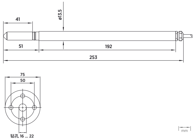
HMP375 探头和不锈钢安装法兰尺寸
