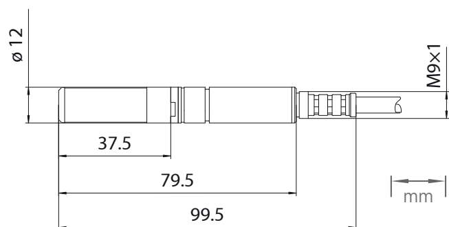
HMP377 尺寸
