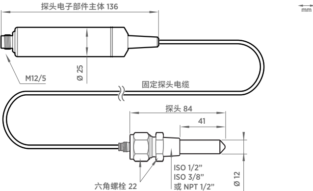
DMP7 尺寸
